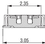
X-X' 断面図
